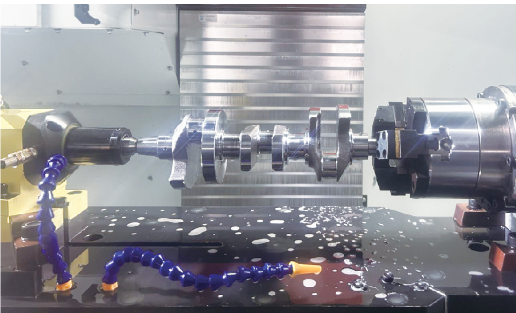
青岛德盛机械制造有限公司为张雪机车装机的曲轴产品。
